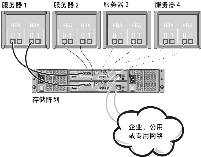
图 2-5. 四台主机连接到两个控制器
