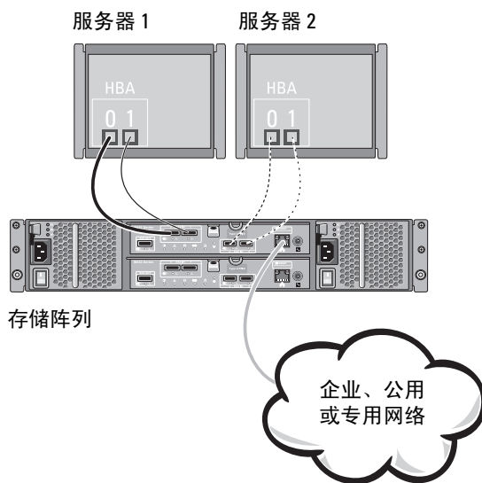
图 2-2. 两台主机连接到单个控制器
