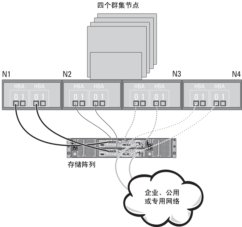
图 2-9. 四个群集节点连接至两台控制器
