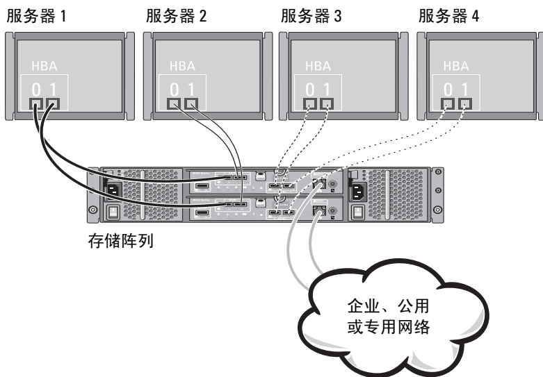
图 2-6. 四台主机连接到两个控制器
