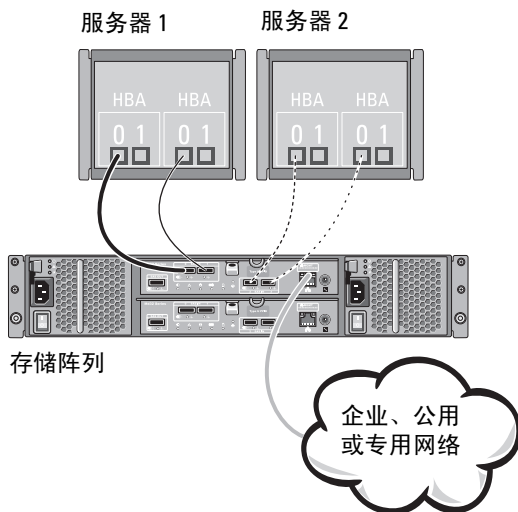
图 2-1. 两台主机连接到单个控制器
