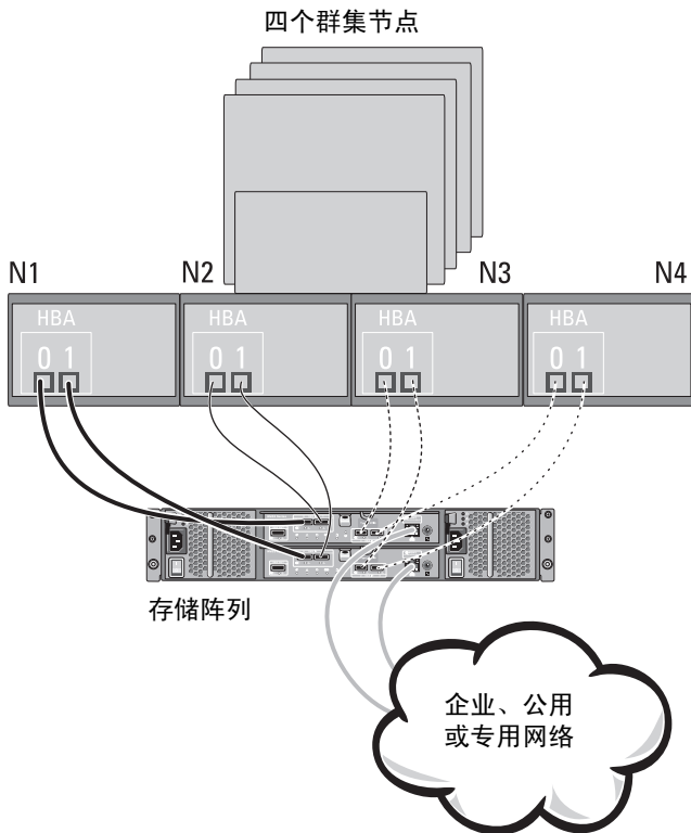
图 2-8. 四个群集节点连接至两台控制器
