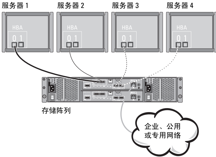
图 2-3. 四台主机连接到单个控制器
