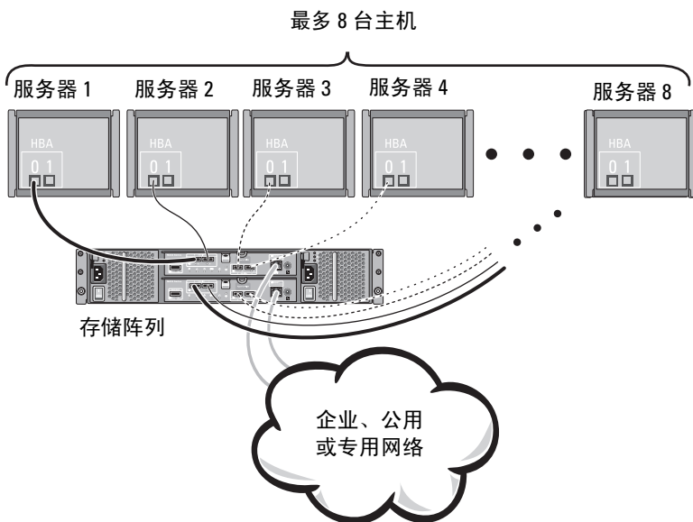
图 2-7. 八台主机连接到两个控制器
