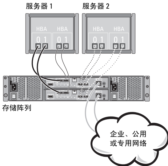
图 2-4. 两台主机连接到两个控制器
